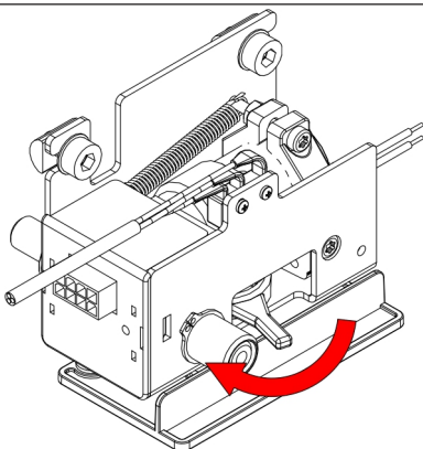
Bei Mehrpunktverriegelung (MPV)
